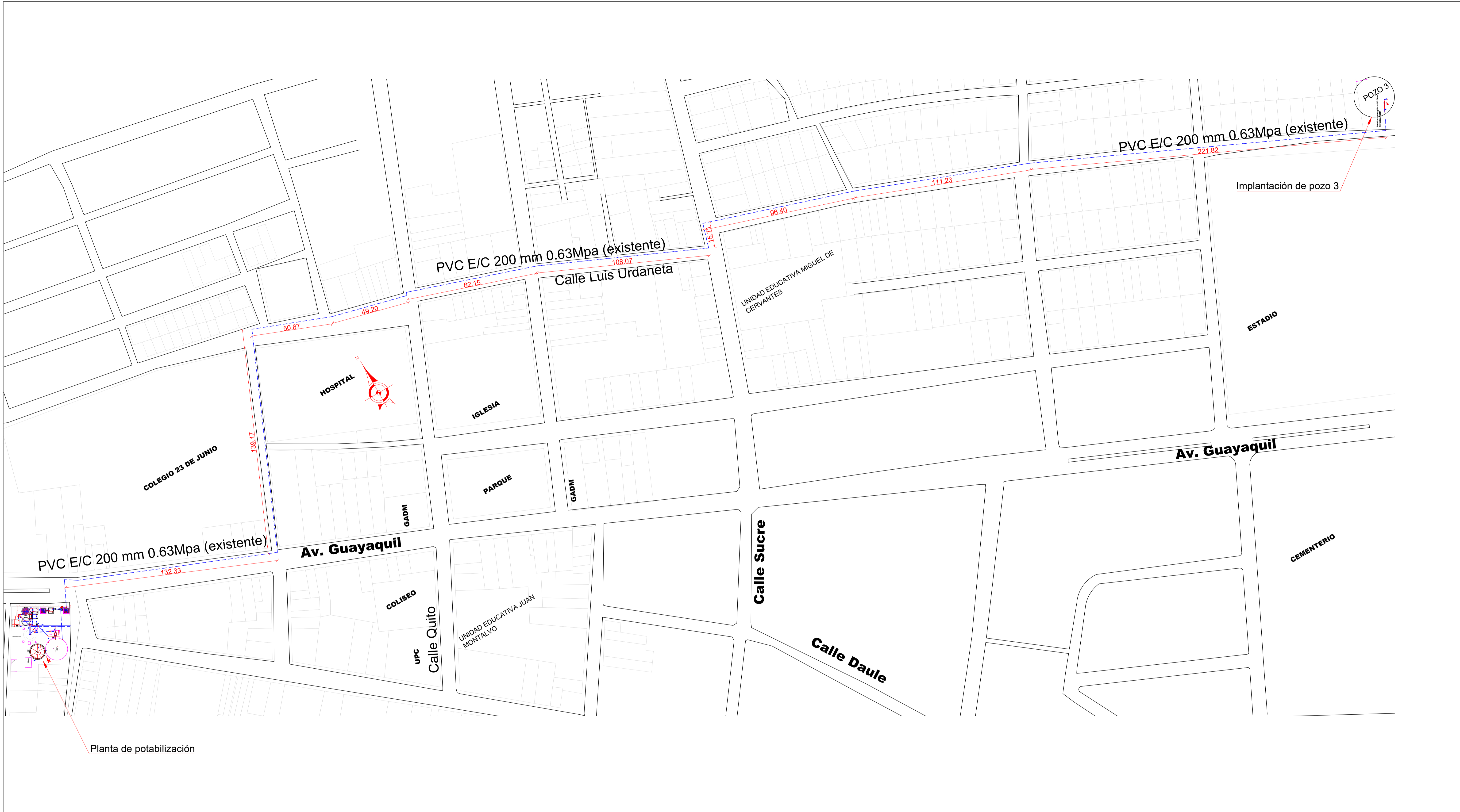
IMPLANTACIÓN GENERAL SISTEMA DE POTABILIZACIÓN DE AGUA DE LA CABECERA CANTONAL DE BABA Escala: _____ 1:1100
